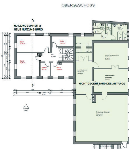
Plan Grundriss OG
