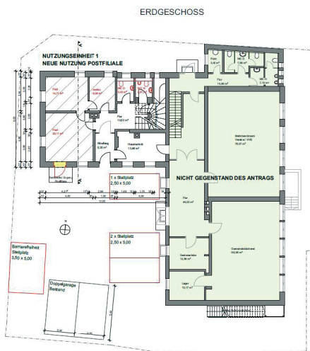
Plan Grundriss EG
