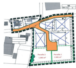
Bebauungsplan „Eresinger Straße“ Ortsteil Ramsach Mischgebiet
